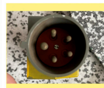
CEF Ausschalter mit Stecker 4,2-6,7A CGBMT516/6h/KA 380 V / 16 A / 50 Hz Art.-Nr.: 19066
