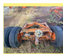
Untersetzachse UN8 Kranfahrwerk, 25 km/h BJ: 1979, Tragkraft 5500 kg Spurweite 1700
