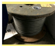
Katzenseil zurück D: 8,00mm 69m für SK96 oder 96/1
