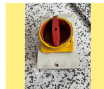
Hauptschalter / Trennschalter für Elektrogeräte Schutzart: IP65
